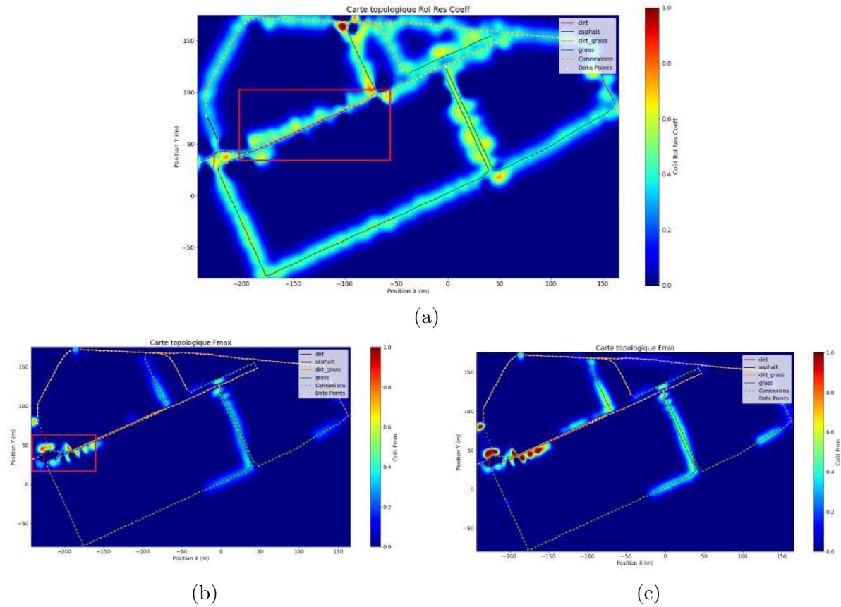
FIGURE 5.10 – Cartes topologiques générée avec le script python pour l'enregistrement de 30 minutes à Verexal : (a) résistance au roulement ; (b) force motrice maximale ; (c) force motrice minimale. Un coût de 0 correspond à un environnement très favorable et un coût de 1 à un environnement très défavorable. Les rectangles rouge sur (a) et (b) correspondent respectivement aux zoom des Figures 5.13 et 5.12.
