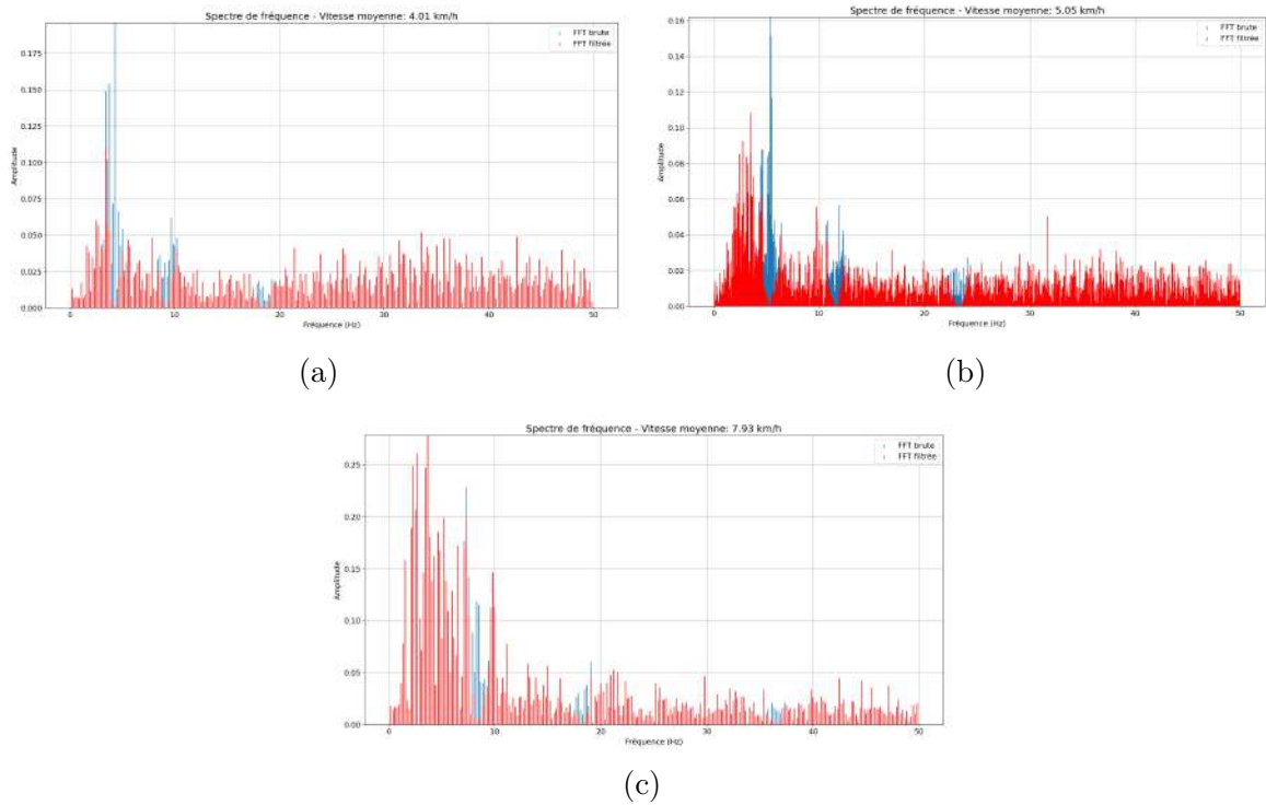
FIGURE 4.24 – Analyse fréquentielle des mesures de l'IMU à (a) 4 km/h, (b) 5 km/h et (c) 8 km/h dans les herbes hautes lors de l'essai 2.
