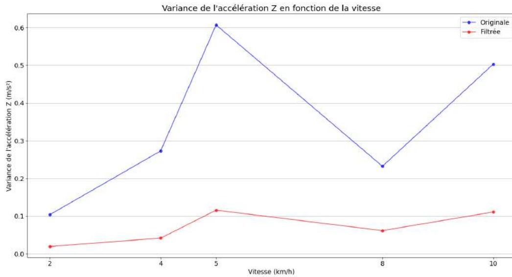
FIGURE 4.25 – Affichage de la variance des mesures de l’IMU en fonction de la vitesse du robot sur l’essai 1.
