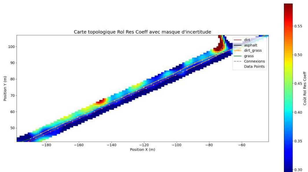
FIGURE 5.13 – Zoom sur la carte topologique de C_{rr} présentée par la Figure 5.10 (a) avec application du masque d'incertitude.
