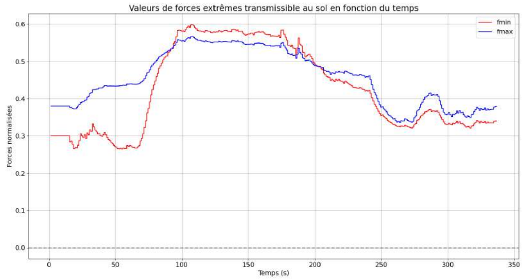
FIGURE 5.4 – Estimations de force motrice maximale et minimale transmissible sur l'essai 3.
