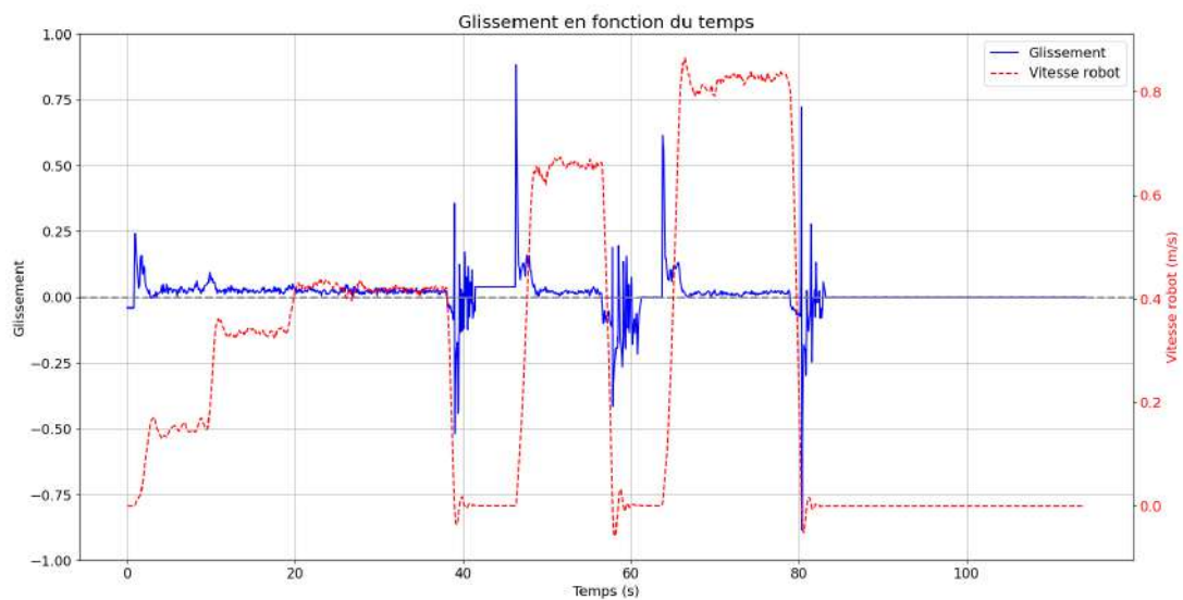
FIGURE 4.9 – Mesures de glissement de l'essai 2.
