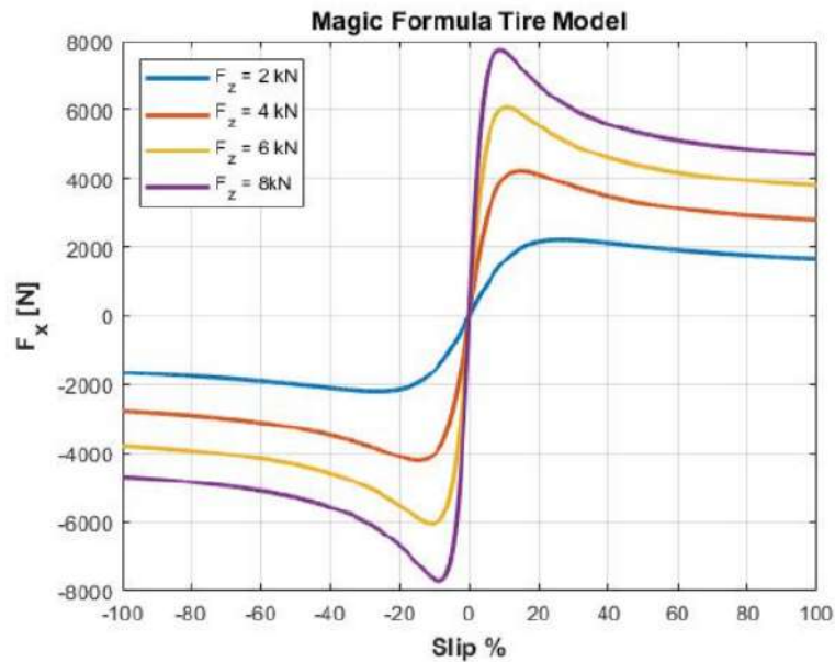
FIGURE 3.1 – Exemple de courbes de force en fonction du glissement extrait de [1]. Ces valeurs sont calculées à l'aide de la magic tyre formula F_x = F_z \cdot D \cdot \sin(C \cdot \arctan(B\mu - E[B\mu - \arctan(B\mu)])) où F_x est la force de traction, F_z la force normale au sol, B , C , D et E sont des coefficients dépendants du type de terrain et de la roue.
