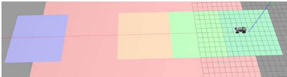
FIGURE 4.4 – Présentation des zones de friction simulées dans Gazebo Classic. Les zones de couleurs vert foncé, vert clair, orange, rouge et bleu correspondent respectivement à des coefficients de friction de 10 (à des fins de debug), 1, 0.5, 0.1 et 0.01.
