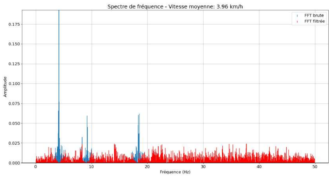
FIGURE 4.21 – Analyse fréquentielle des mesures de l’IMU à 4 km/h sur de l’asphalte lors de l’essai 1.
