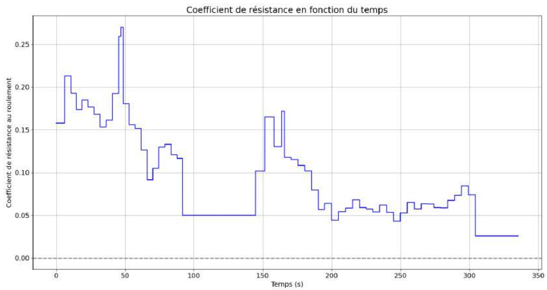
FIGURE 4.12 – Coefficient de résistance au roulement de l'essai 3.
