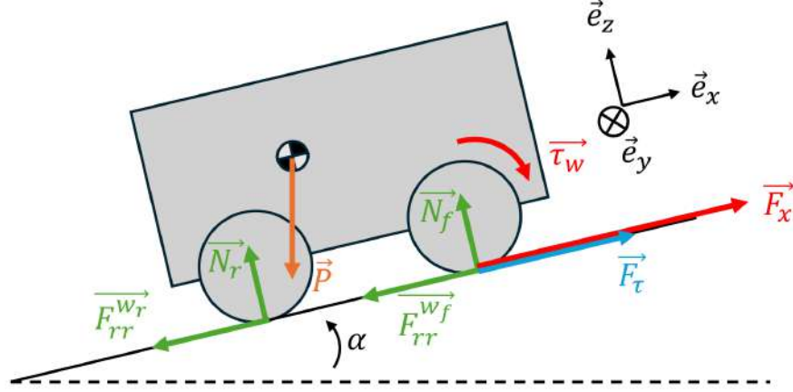
FIGURE 3.3 – Schéma des forces agissant sur le robot. \vec{P} représente le poids du robot, \vec{\tau}_w le couple au niveau des roues, \vec{F}_x la force motrice du robot, \vec{F}_{rr}^{wf} et \vec{F}_{rr}^{wr} sont respectivement les forces de résistance au roulement des roues avant et arrière, \vec{N}_f et \vec{N}_r les forces normales au sol pour les roues avant et arrière, \vec{F}_\tau la force motrice efficace du robot et \alpha l'angle de la pente du terrain. Le repère du robot est noté \vec{e}_x, \vec{e}_y, \vec{e}_z .
