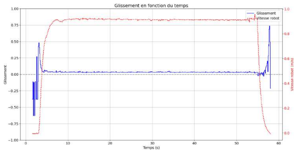
FIGURE 4.6 – Essais à vitesse constante sur les cinq zones de friction simulées dans Gazebo Classic.
