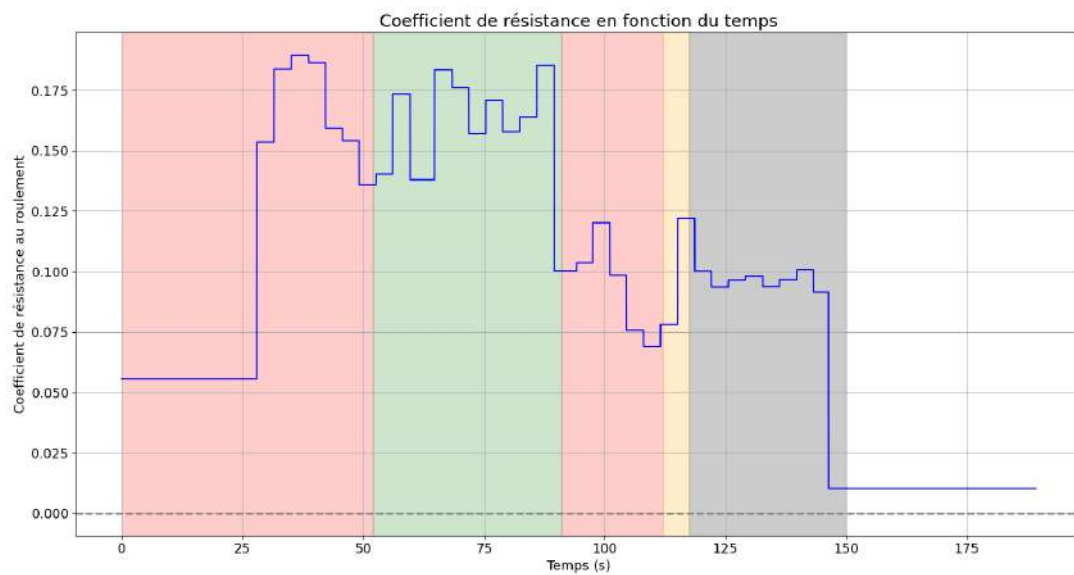
FIGURE 4.13 – Coefficient de résistance au roulement de l'essai 7. Les couleurs de fond indiquent le type de terrain traversé : rouge, mélange terre et herbe ; vert, herbes hautes ; orange, terre ; gris, asphalte.
