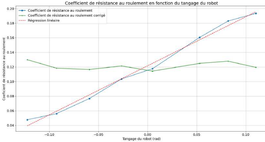
FIGURE 4.15 – Résultat de la régression linéaire pour calculer l’invariant de pente sur l’essai 3.
