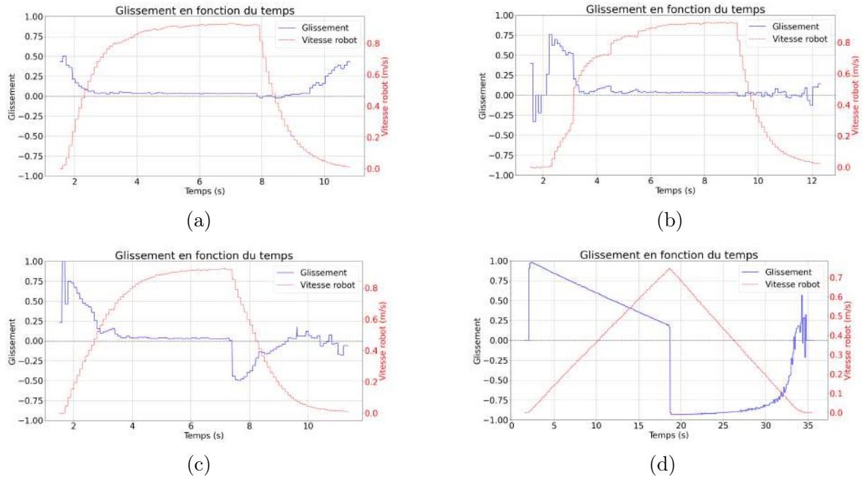
FIGURE 4.5 – Essais en phase d’accélération et de décélération sur les différentes zones de friction simulées dans Gazebo Classic. (a) zone de haute friction, (b) zone de friction moyenne, (c) zone de faible friction, (d) zone de très faible friction.
