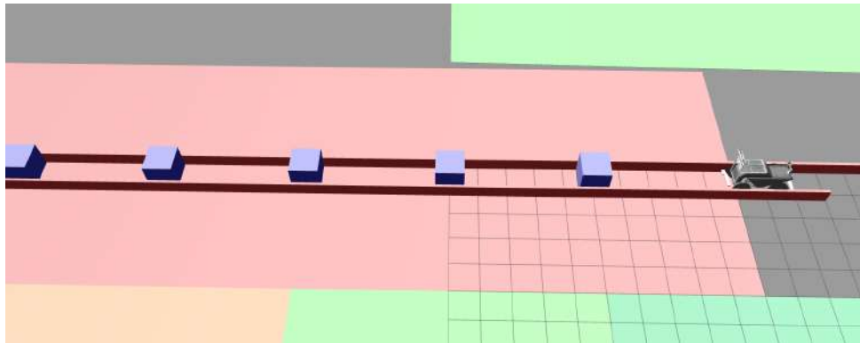
FIGURE 4.7 – Présentation du setup de mesure de glissement dans Gazebo Classic.
