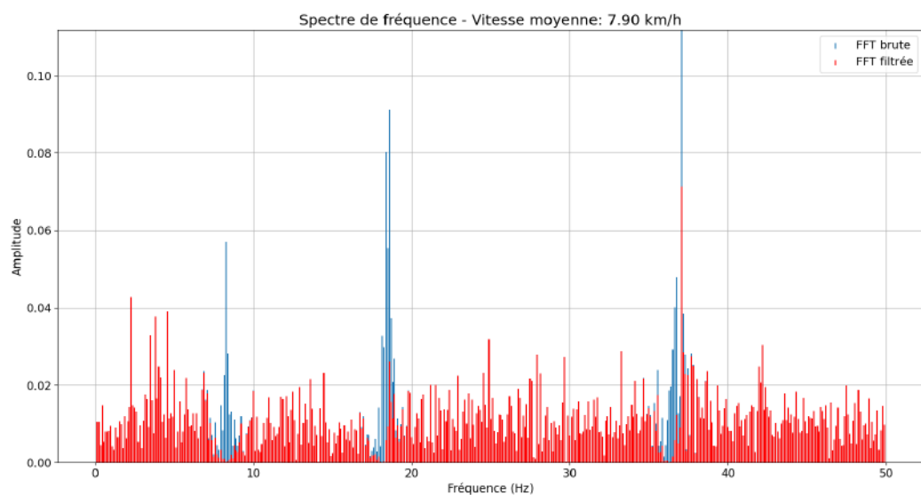
FIGURE 4.23 – Analyse fréquentielle des mesures de l’IMU à 8 km/h sur de l’asphalte lors de l’essai 1.
