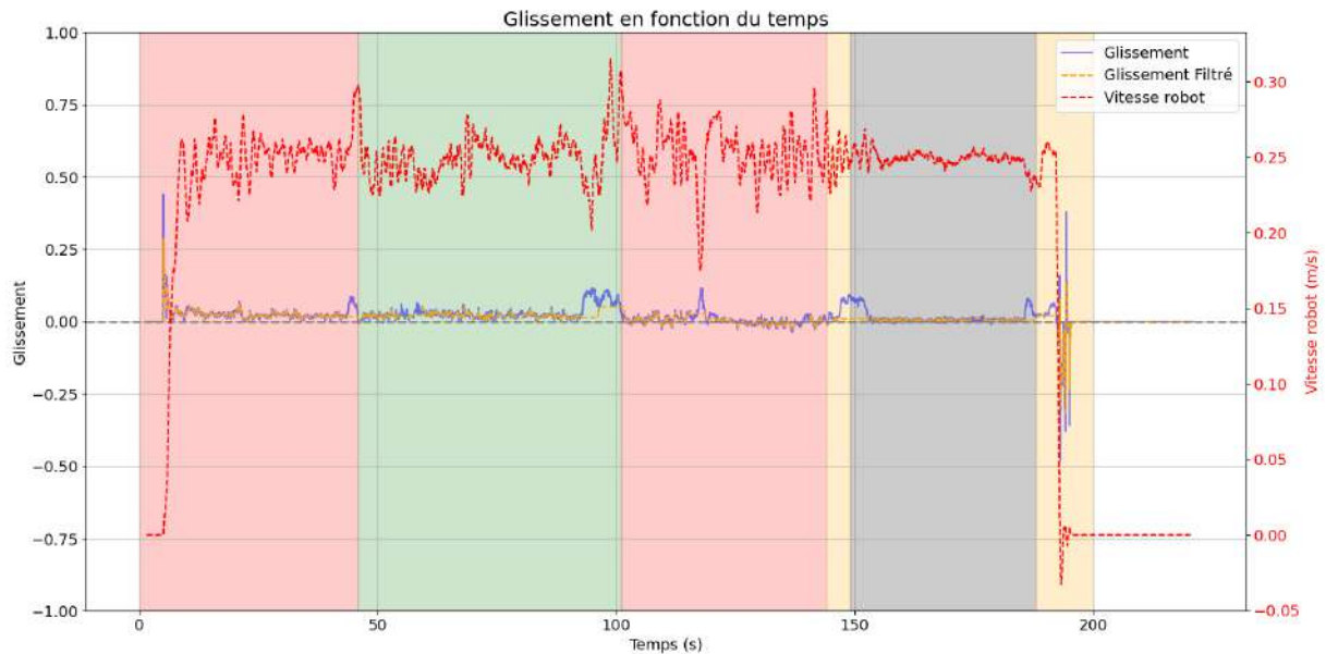
FIGURE 5.3 – Calculs de glissement réalisées sur le rosbag de l’essai 6. Les couleurs de fond indiquent le type de terrain traversé : rouge, mélange terre et herbe ; vert : herbes hautes ; orange : terre ; gris : asphalte.
