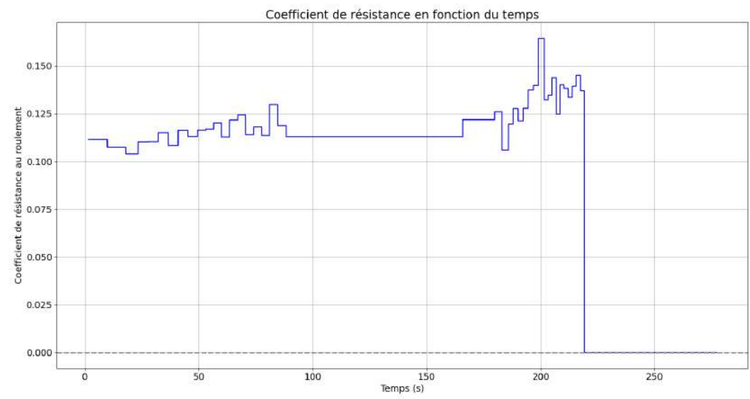
FIGURE 5.8 – Coefficient de résistance au roulement sur le rosbag de l’essai 9.
