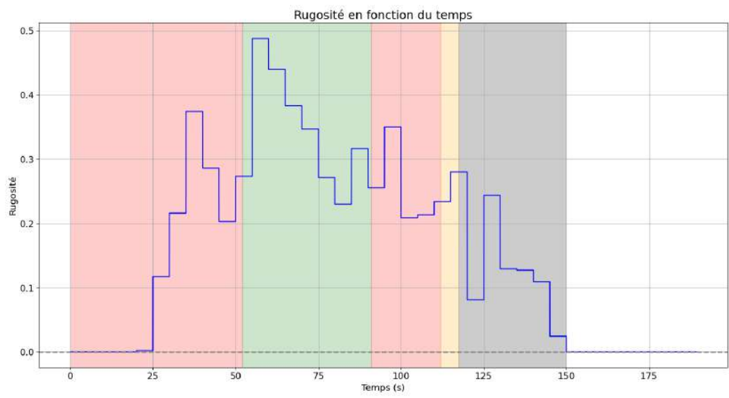
FIGURE 4.20 – Résultats de rugosité pour l’essai 7. Les couleurs de fond indiquent le type de terrain traversé : rouge, mélange terre et herbe ; vert, herbes hautes ; orange, terre ; gris, asphalte.
