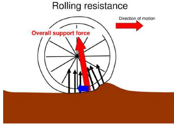
FIGURE 3.2 – Schéma décrivant la résistance au roulement
