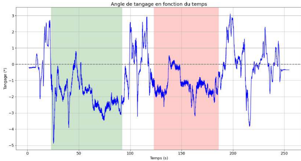
FIGURE 5.9 – Mesure du tangage de KIPP pour l’essai sur le parking de l’Englab. La zone marquée en vert correspond à l’aller et la zone en rouge au retour.
