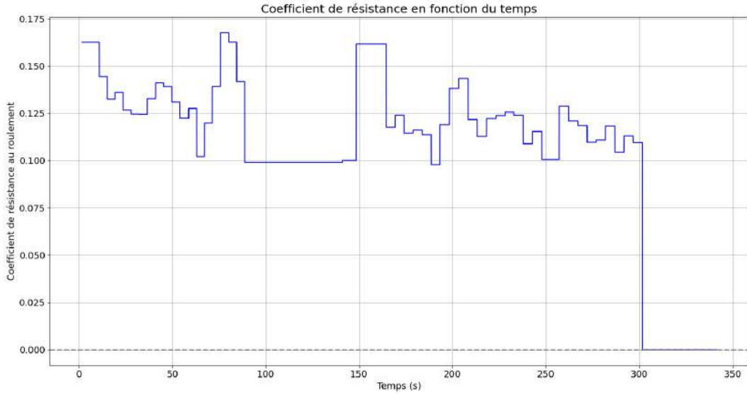
FIGURE 5.6 – Coefficient de résistance au roulement sur le rosbag de l’essai 3.
