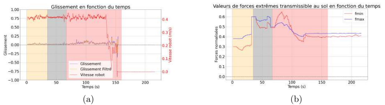
FIGURE A.20 – Résultats de (a) glissement et de (b) forces extrêmes transmissibles pour le long enregistrement à Verexal. Les couleurs de fond correspondent aux terrains traversés. Rouge : mélange herbe et terre ; orange : terre ; gris : asphalte.
