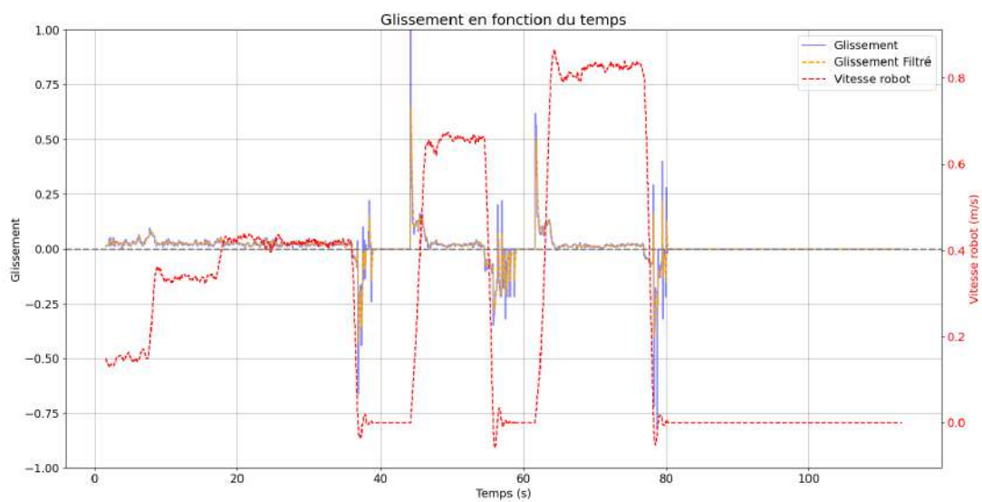
FIGURE 5.2 – Calcul de glissement sur le rosbag de l'essai 2.
