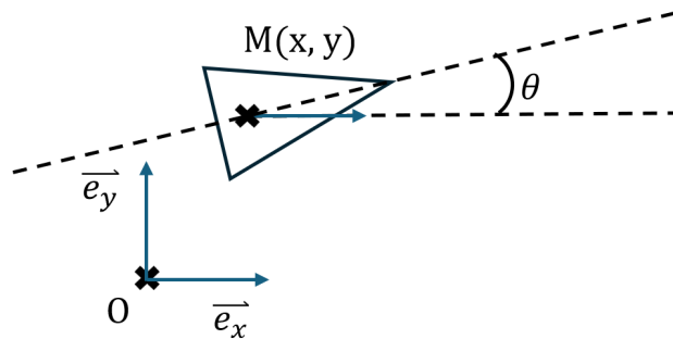
Figure 1 – Représentation de l'état d'une base mobile
