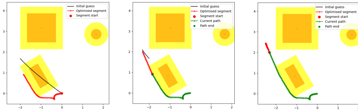
Figure 10 – Fonctionnement de l’horizon adaptatif utilisé par la méthode des optimisations adjacentes (axes gradués en mètres)
