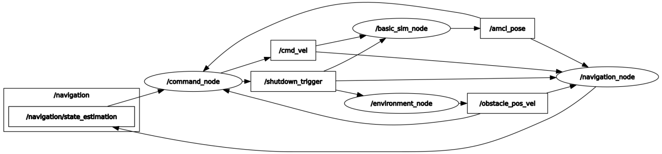
Figure 4 – Graphe des nœuds et topics du paquet ROS2
