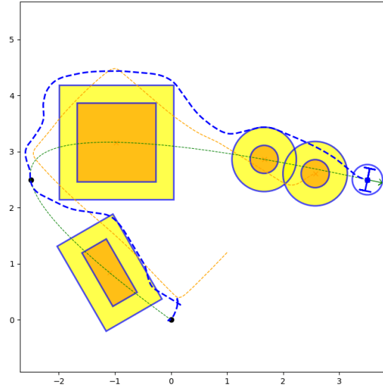
Figure 7 – Trace obtenue pour l'évitement d'obstacles dynamiques basé sur le contrôleur MPC (axes gradués en mètres)
