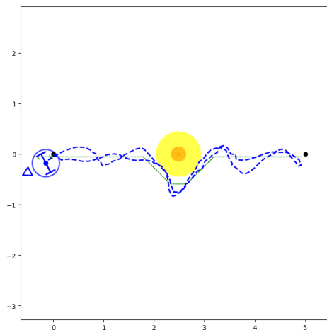
Figure 8 – Traces obtenue pour l'évitement d'obstacles statiques en condition réelles (axes gradués en mètres)
