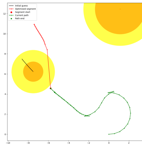
Figure 9 – Exemple d'horizon de prédiction invalide pour la méthode des optimisations adjacentes
