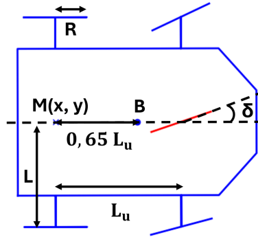
Figure 2 – Représentation géométrique d'une base mobile de type Ackermann
