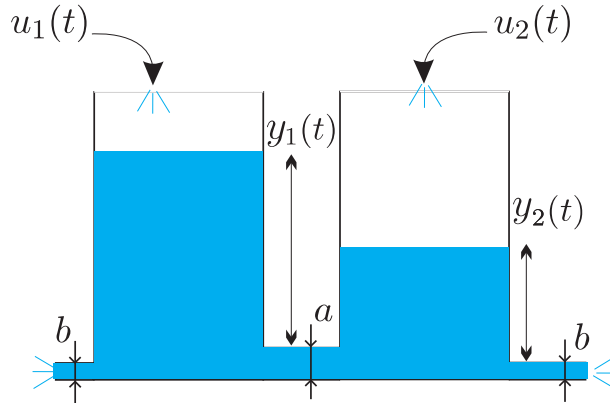
Figure 1. Système hydraulique formé de deux bacs remplis d'eau reliés par un canal.
